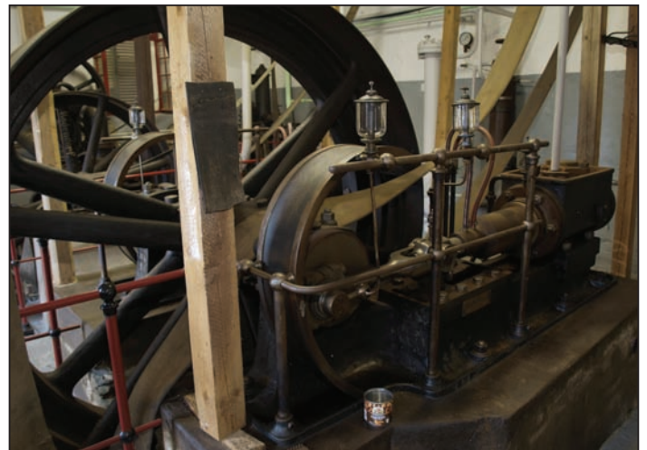
Verdichter mit Transmission Foto: Wolfgang Seidenfuß
